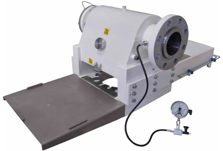
Головка для коротких макаронных изделий
